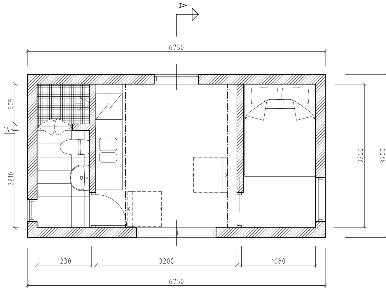
PLAN, NEDRE SKALA 1:50 (A4)
