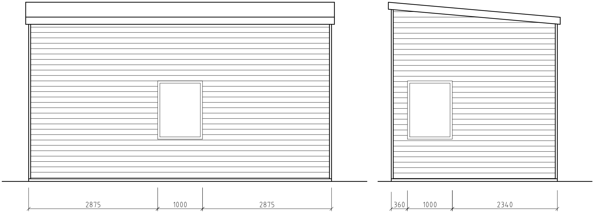
FASADER: BAKSIDA + GAVEL SKALA 1:50 (A4)
