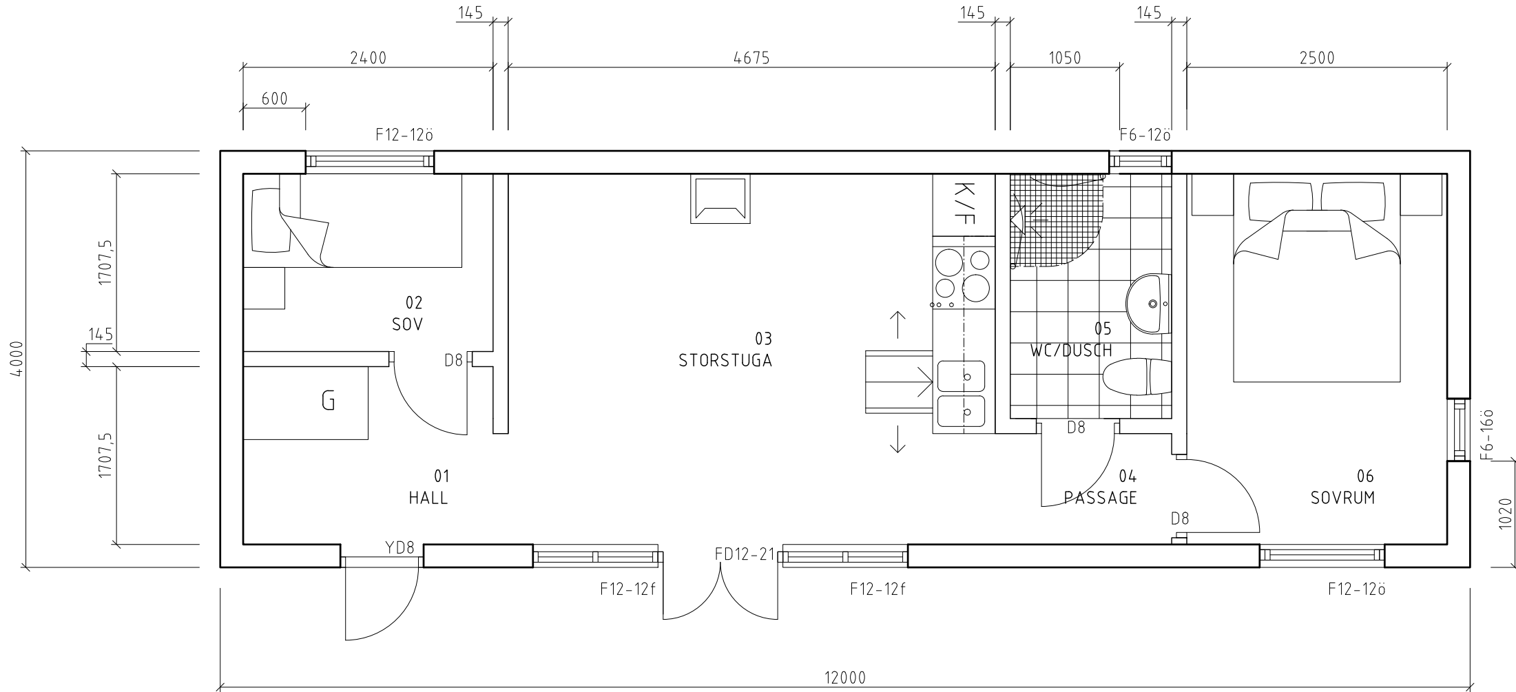
PLANSKISS SKALA 1:50 (A4)
